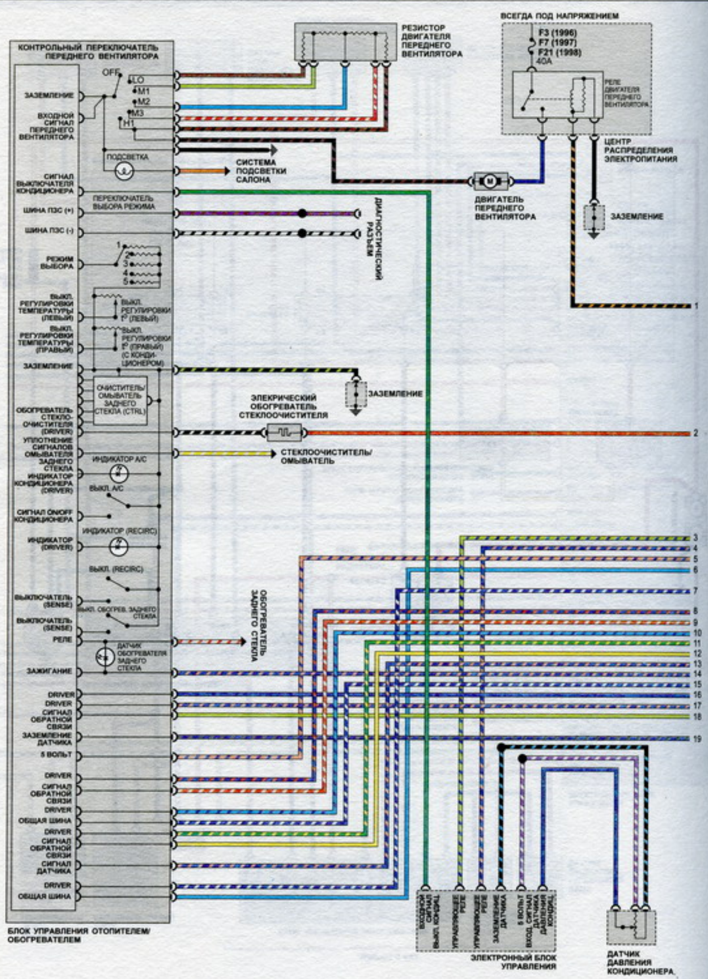
5. Кондиционер и отопитель - включая вентилятор системы охлаждения (1 из 2)
